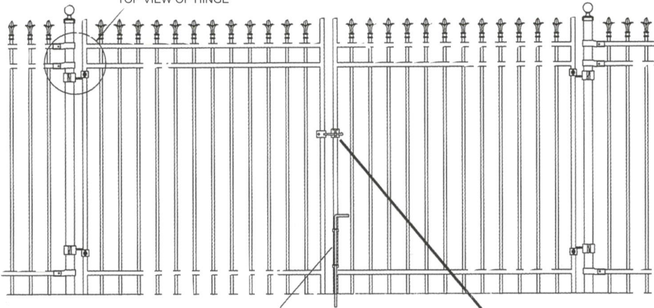
VERROU À BEC-DE-CANE CANE BOLT
